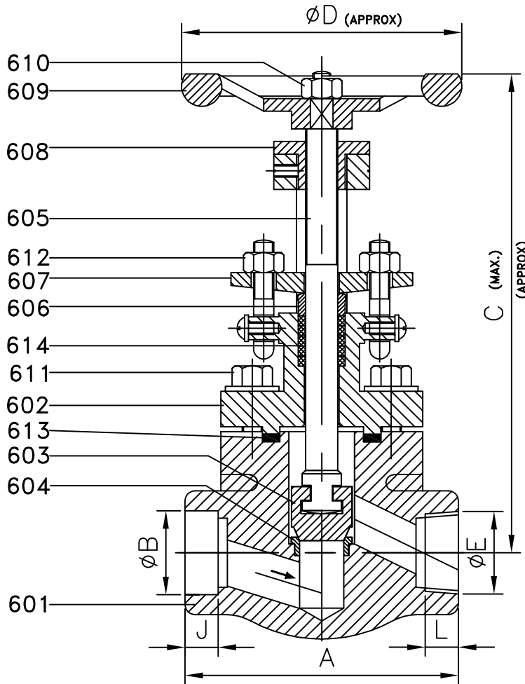
DIMENSION TABLE 1500#
